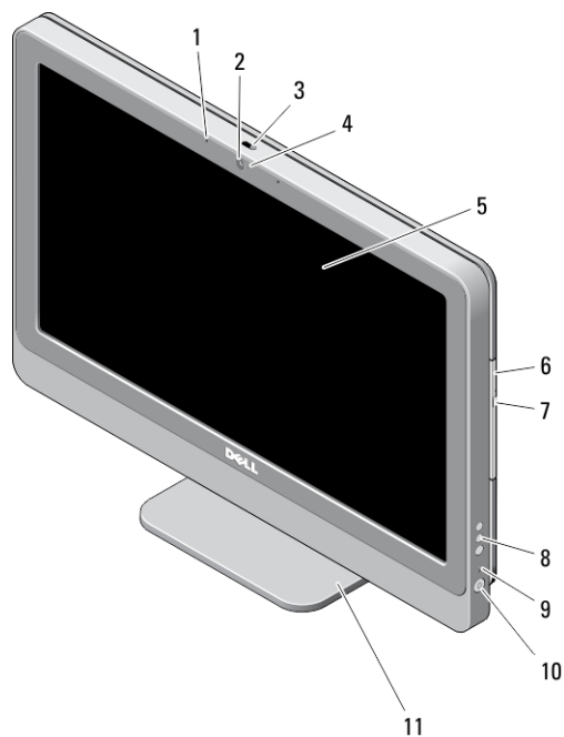
Figura 1. Vista frontal
